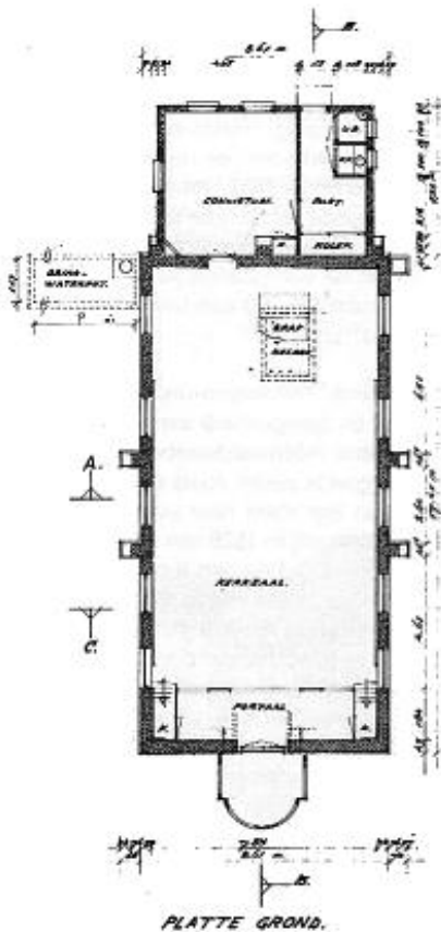
Platte grond.
