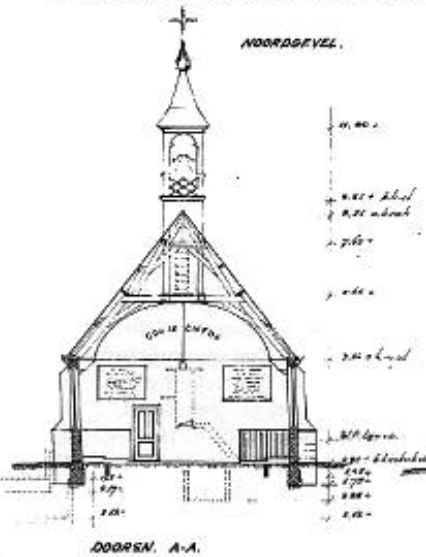
Ooeten A-A.
