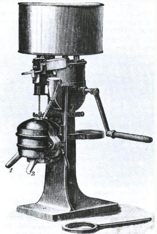
1. Een Mélotte-centrifuge. Dergelijke apparaten vervingen op het eind van de 19e eeuw de grote platte afroombakken en bespoedigen het afroom proces van de melk aanzienlijk.
